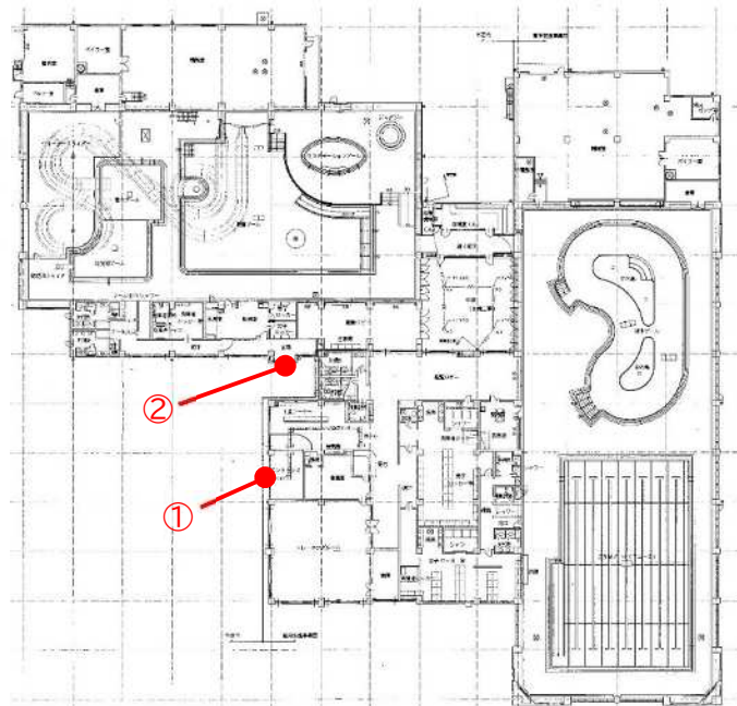
建物内配置図
