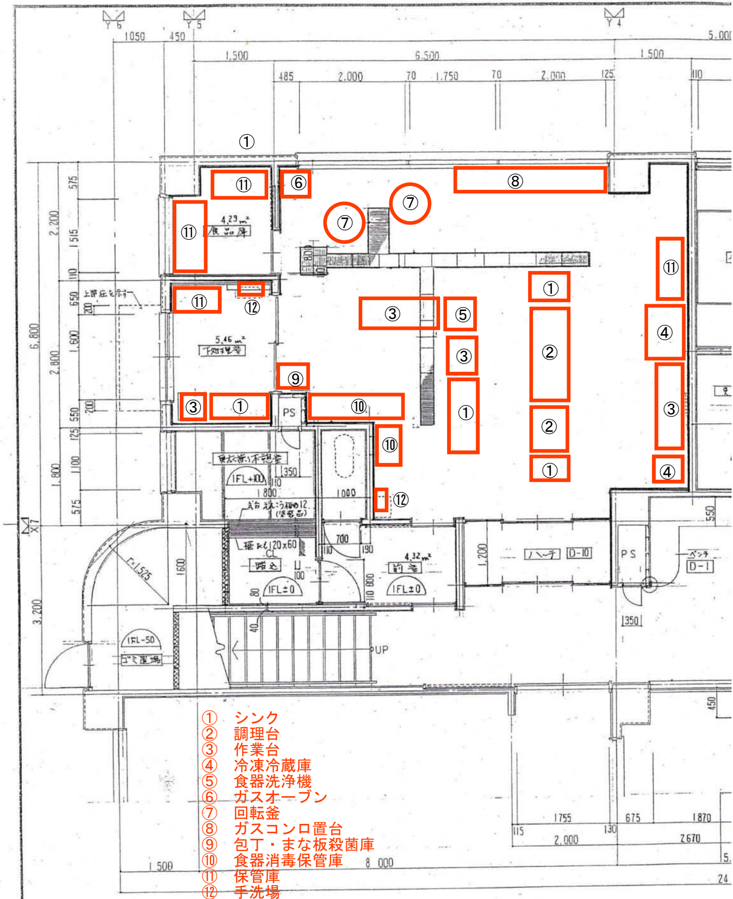
つくし学園調理室設備配置図
