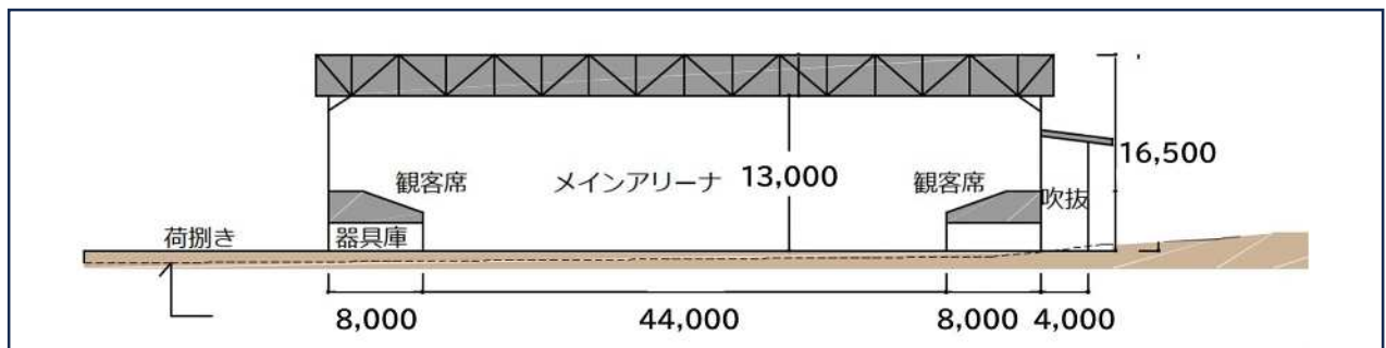
〈断面イメージ図〉
