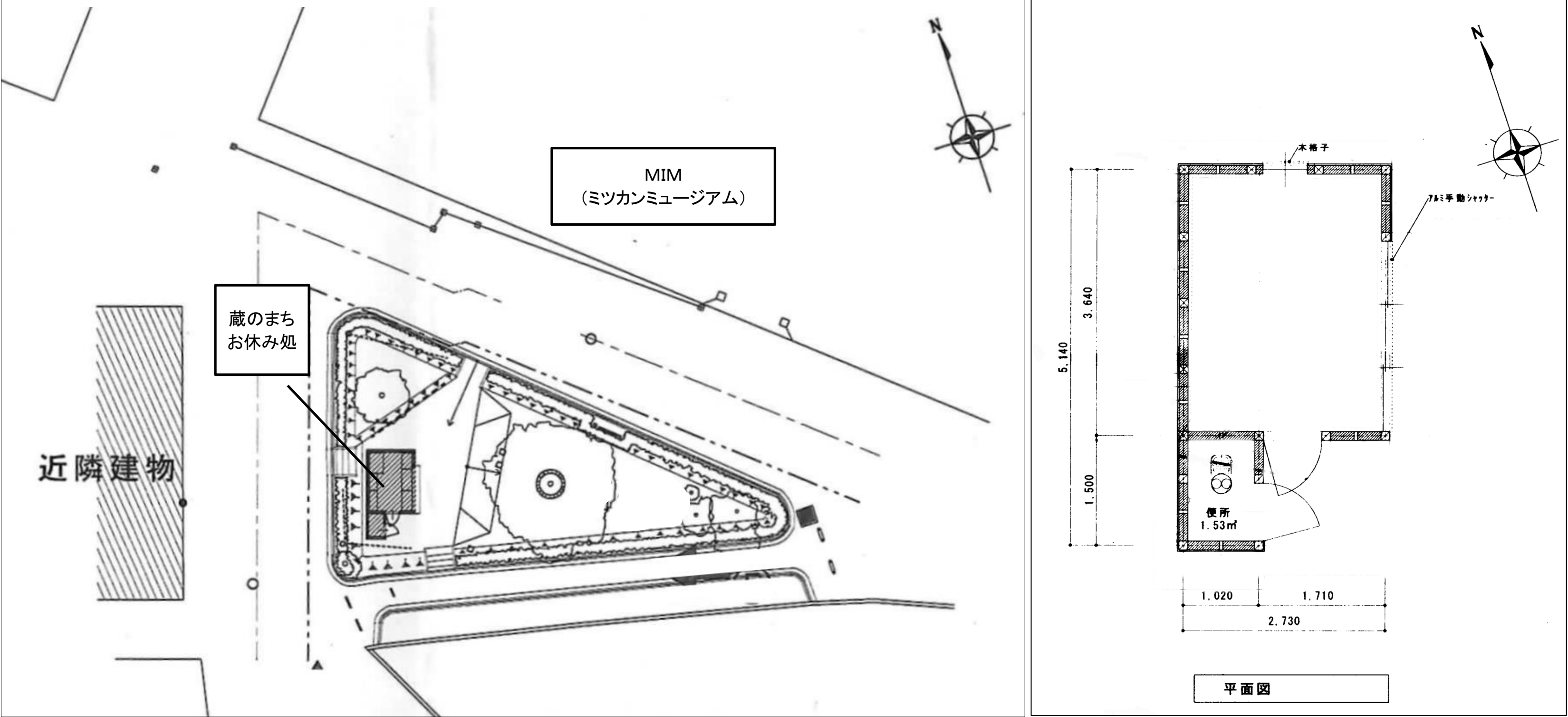
平面図：蔵のまちお休み処（中村街園）
