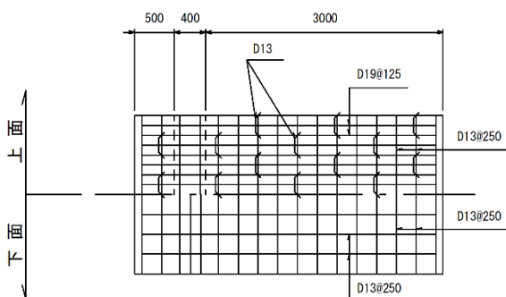
底版配筋図
