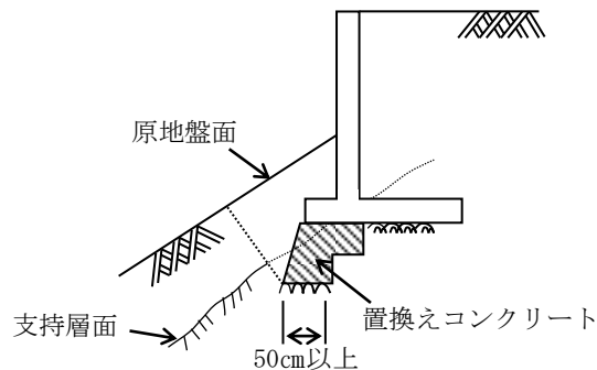
図 5-32 置換えコンクリート上の直接基礎の例
