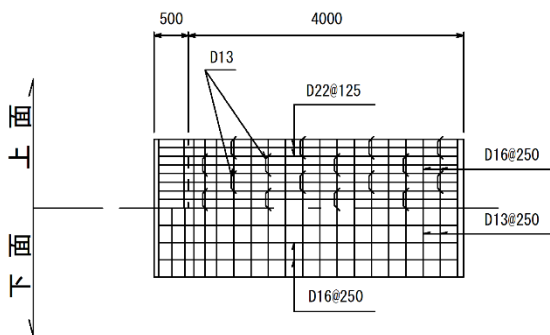
底版配筋図
