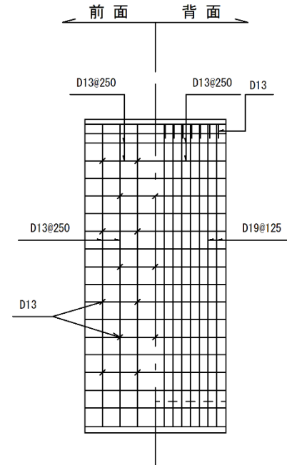
縦壁配筋図
