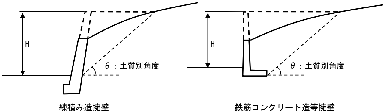
図 5-6 上部に斜面がある場合の擁壁の高さの設定方法
