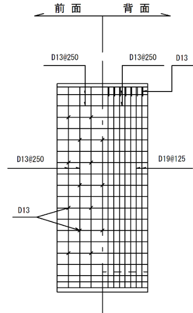
縦壁配筋図
