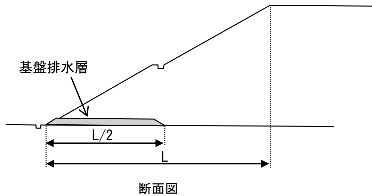
図 2 - 4 基盤排水層の例
