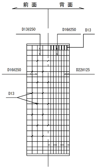
縦壁配筋図
