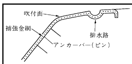
図4-2 吹付工ののり肩部の処理
