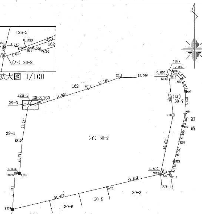
地積測量図
