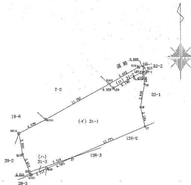
杭標示
