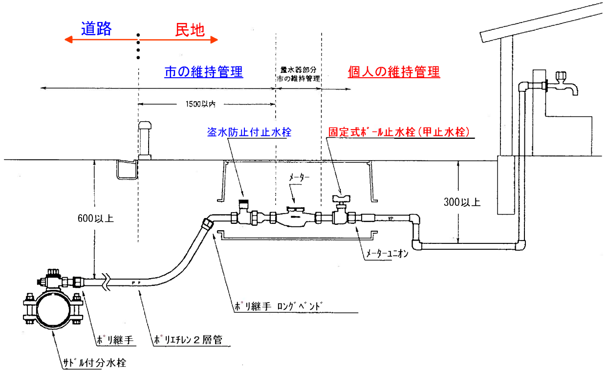
口径25mm以下の標準配管、維持管理図
