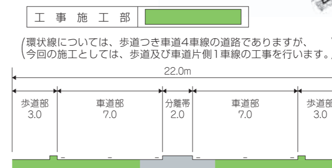
※都市計画道路環状線の道路標準断面図
