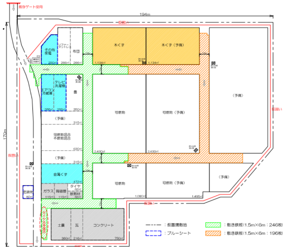
図6 一次仮置場レイアウト例
