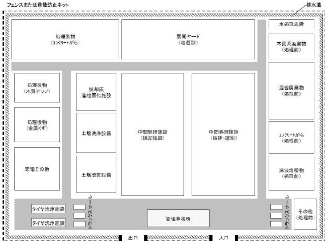
図7 二次仮置場レイアウト例
