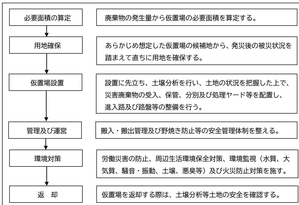
図5 仮置場の設置手順
