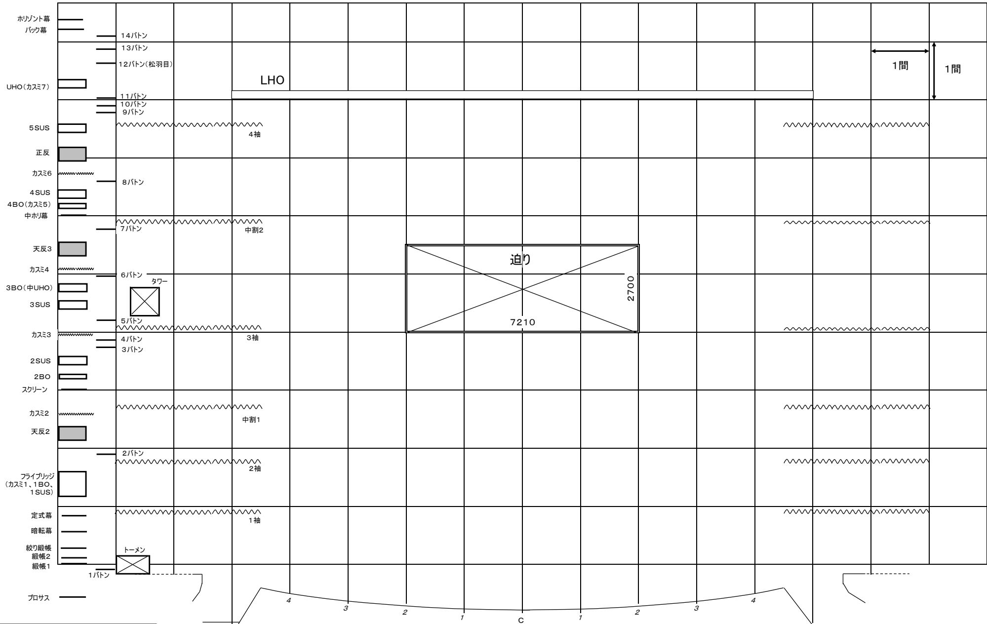
半田市福祉文化会館 瀧上工業雁宿ホール 舞台平面図
