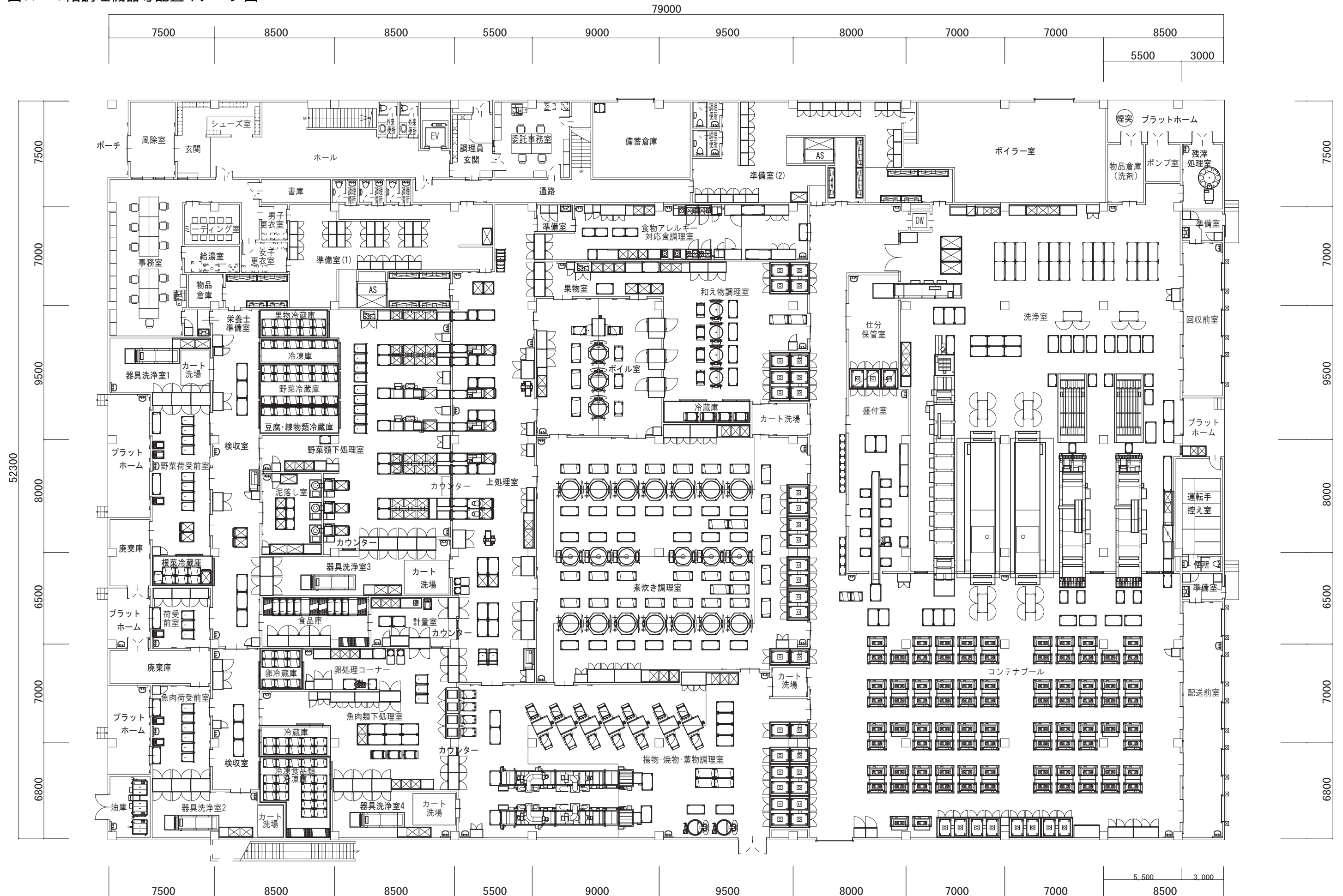
図11 1階調理機器等配置イメージ図
